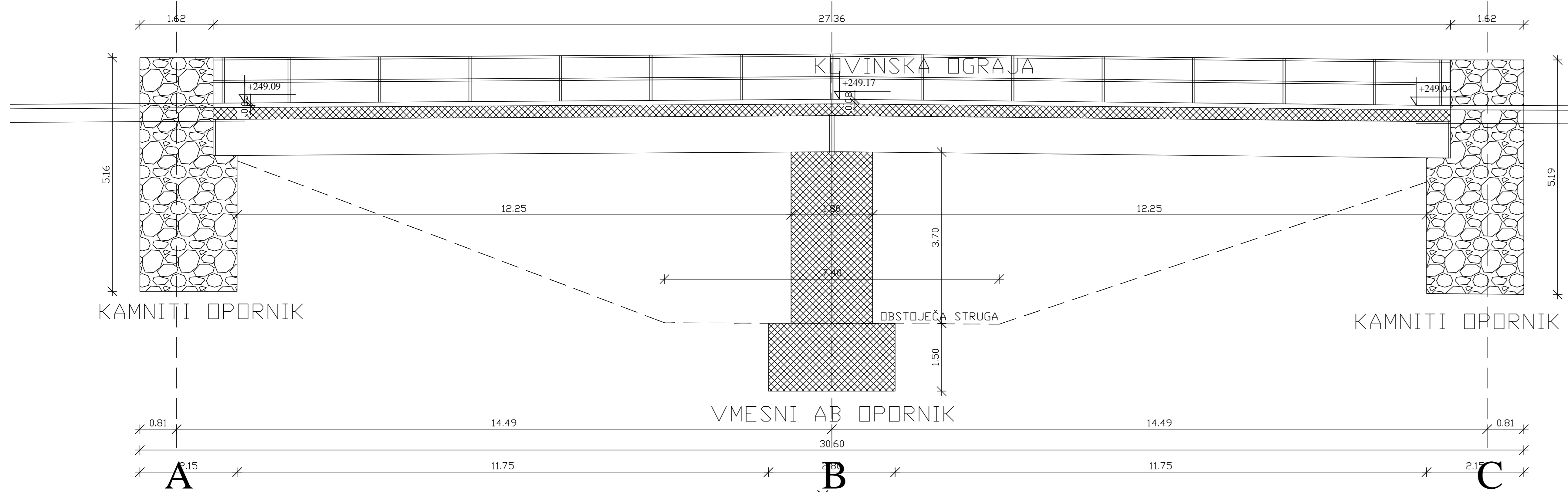
VZDOLŽNI PREREZ
